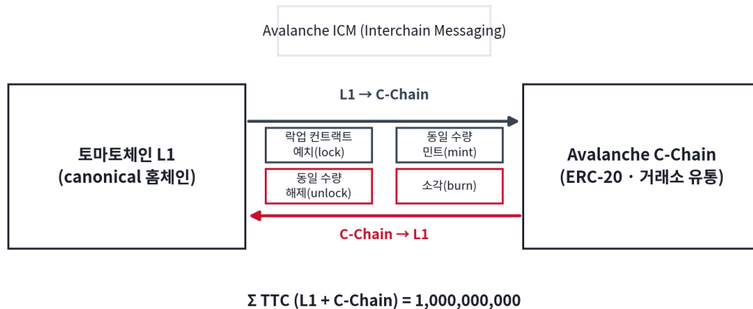
그림 2. 토마토체인 L1 ↔ 아발란체 C-Chain 간 ICM 기반 양방향 이동 (lock-and-mint / burn-and-unlock)
